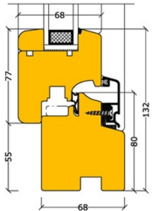
SEZIONE 2
