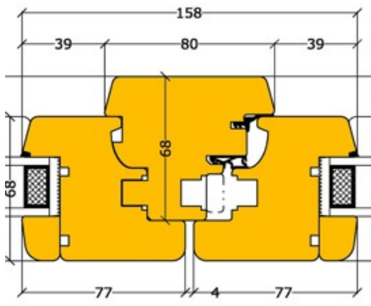
SEZIONE 3
